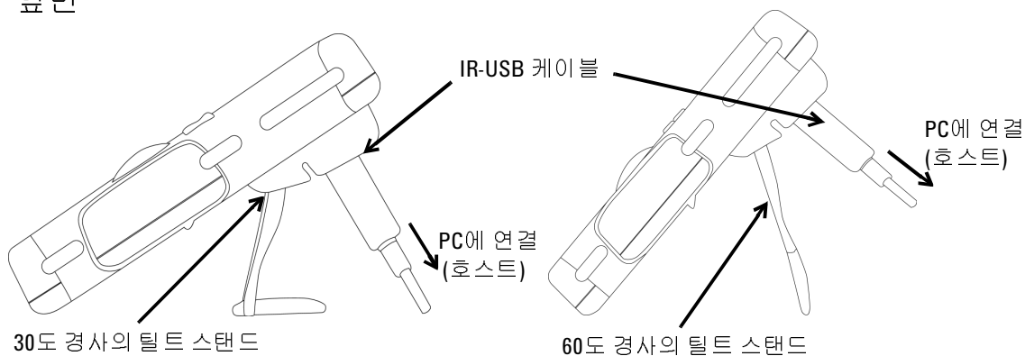
옆면
