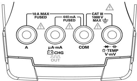
图 1 U1252A 端子
