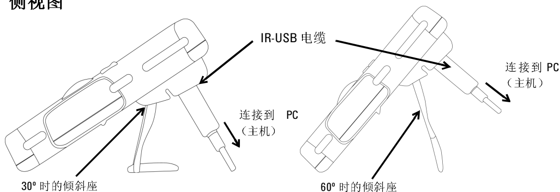
侧视图
