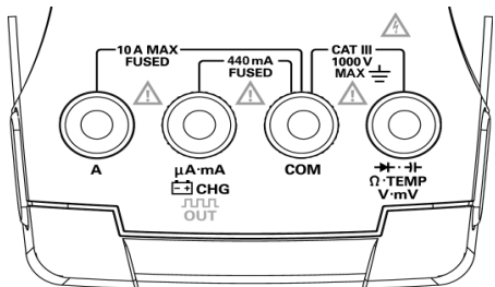
Figura 1 Terminali U1252A
