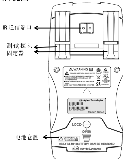
后视图
