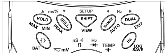
그림 4 U1252A 키패드
