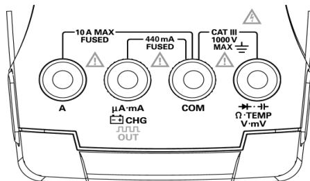
図1 U1252Aの端子
