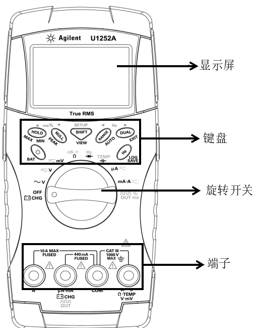
前视图
