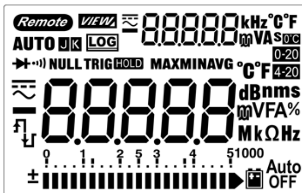
Abbildung 2 Vollständige U1252A-Anzeige
