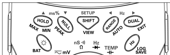
Figura 4 Tastierino U1252A
