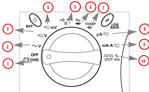
Abbildung 3 U1252A-Drehregler
